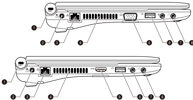
Afbeelding 2-2 Linkerkant van de computer
