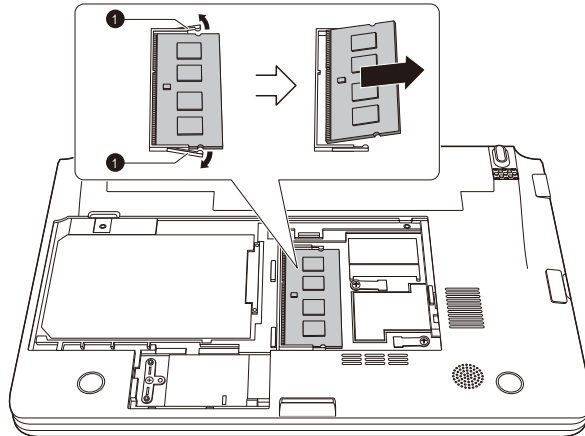
Afbeelding 3-14 De geheugenmodule verwijderen
