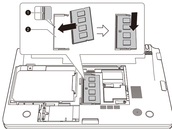
Afbeelding 3-12 De geheugenmodule plaatsen
