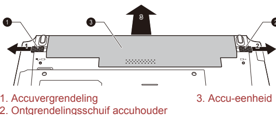
Afbeelding 5-1 De accu-eenheid vrijgeven
