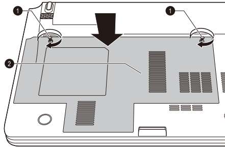
Afbeelding 3-13 Het afdekplaatje over de geheugenmodule plaatsen
