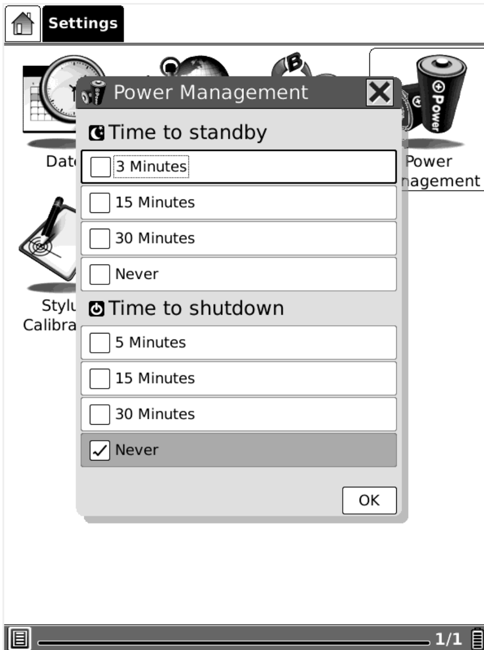
Fig. 6.1.5.4 Dialoogvenster energiebeheer
