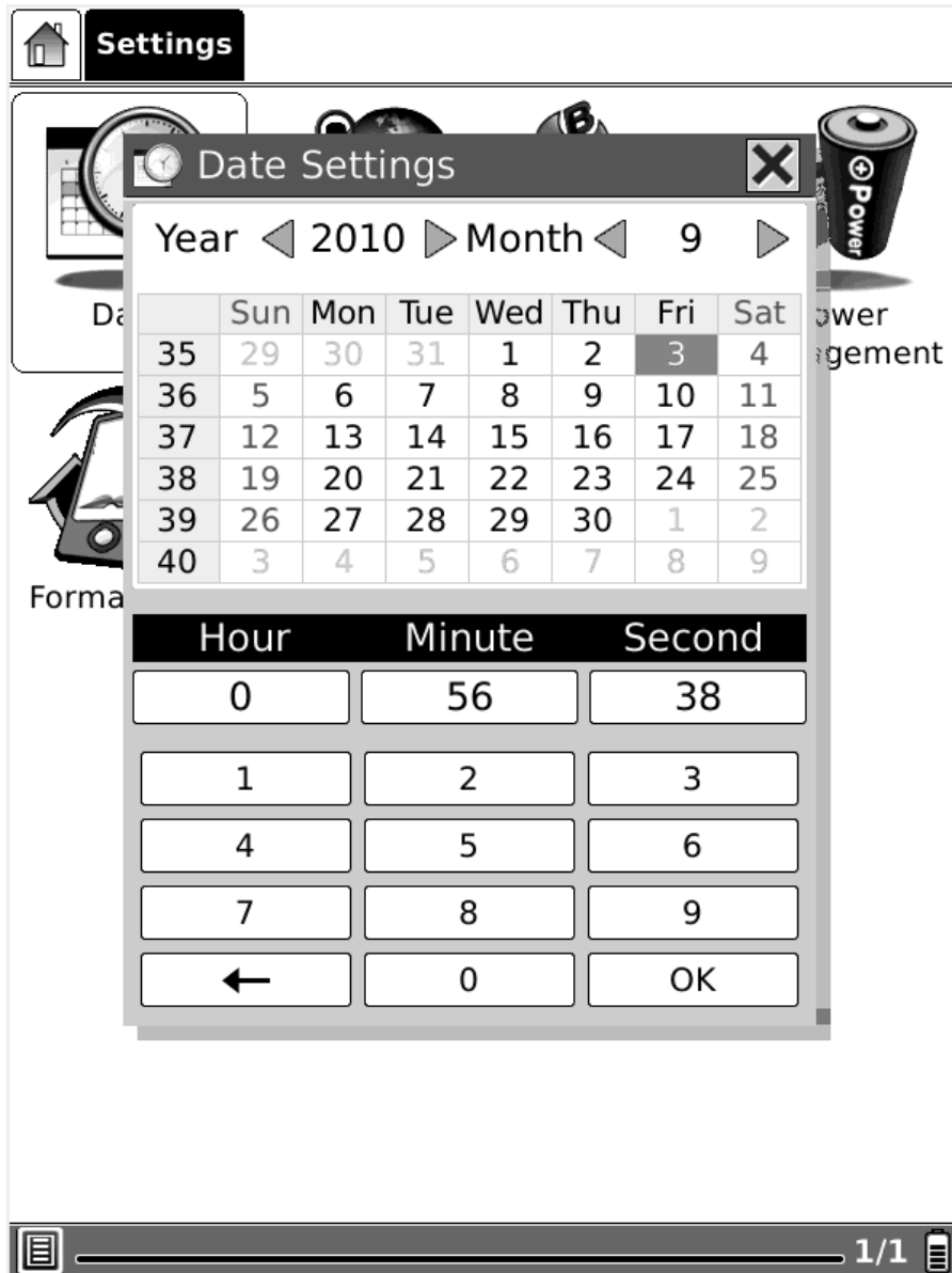
Fig. 6.1.5.1 Dialoogvenster Gegevensconfiguratie
