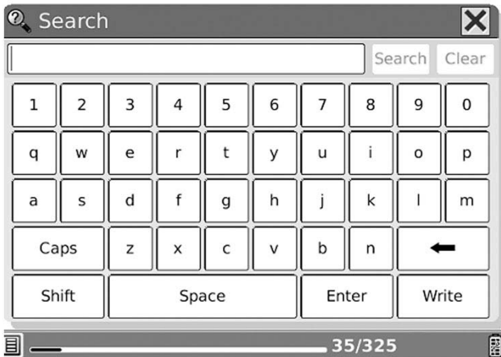
Fig. 6.4.13.1 (1) Zoekpatroon invoeren
