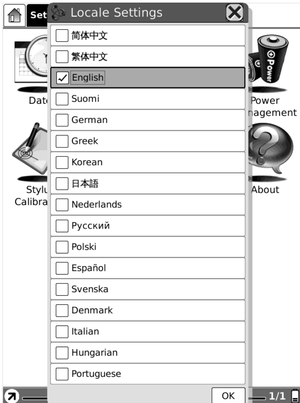
Fig. 6.1.5.3 Dialoogvenster Locale
