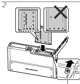
Botón de bloqueo de la batería
